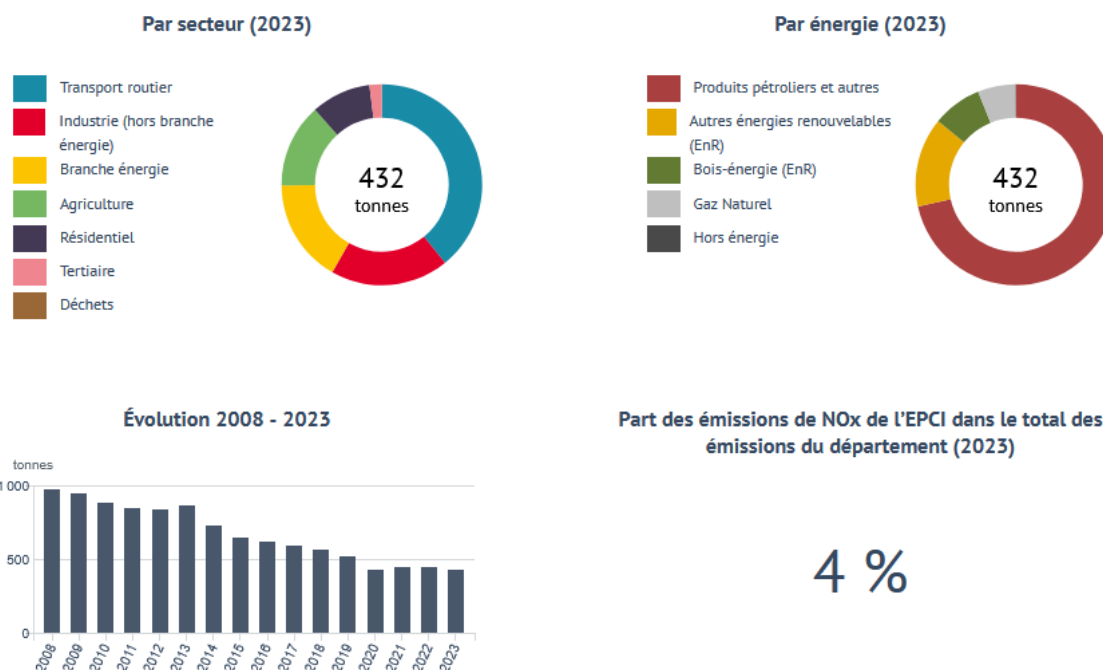
Figure 71 : Bilan des émissions de NOx sur la CC Châteaubriant-Derval en 2023. Source : Air Pays de la Loire
