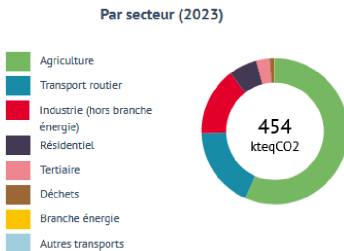
Figure 87 : Emissions des GES en kteqCO2 par secteur en 2023 sur la CC Châteaubriant-Derval. Source : Air Pays de la Loire
