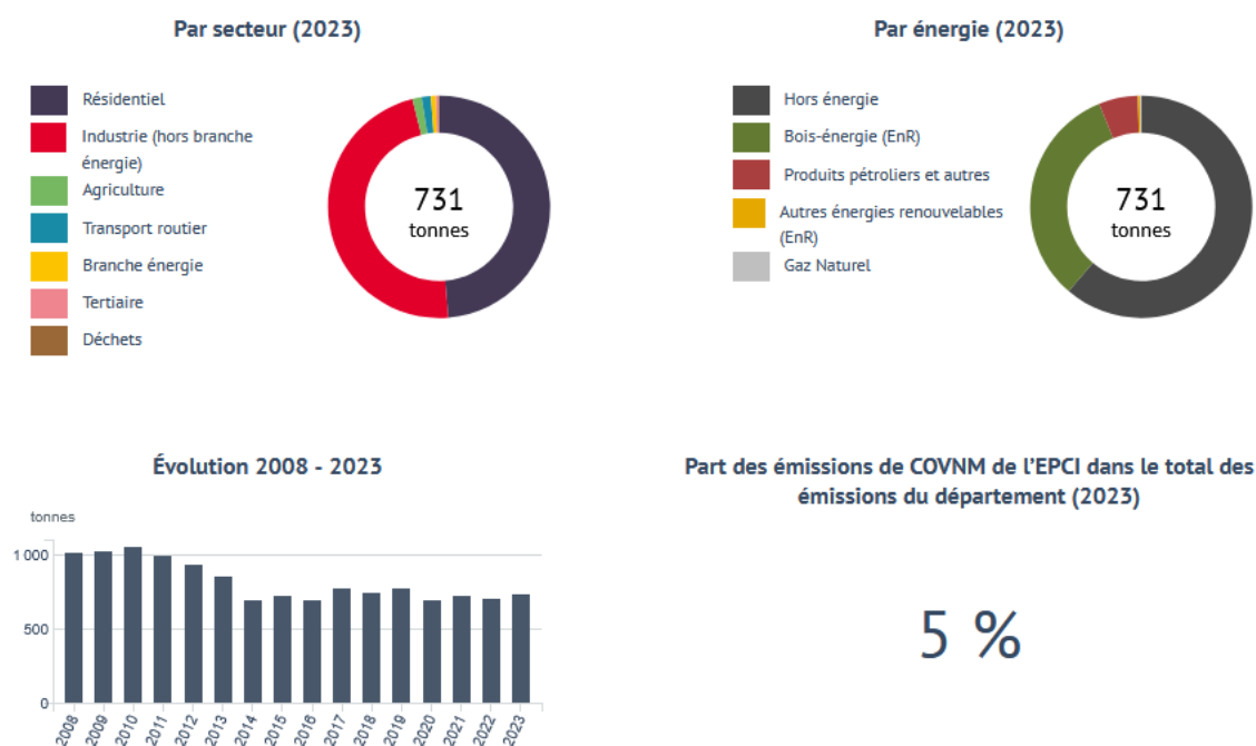
Figure 74 : Bilan des émissions de COVNM sur la CC Châteaubriant-Derval en 2023. Source : Air Pays de la Loire
