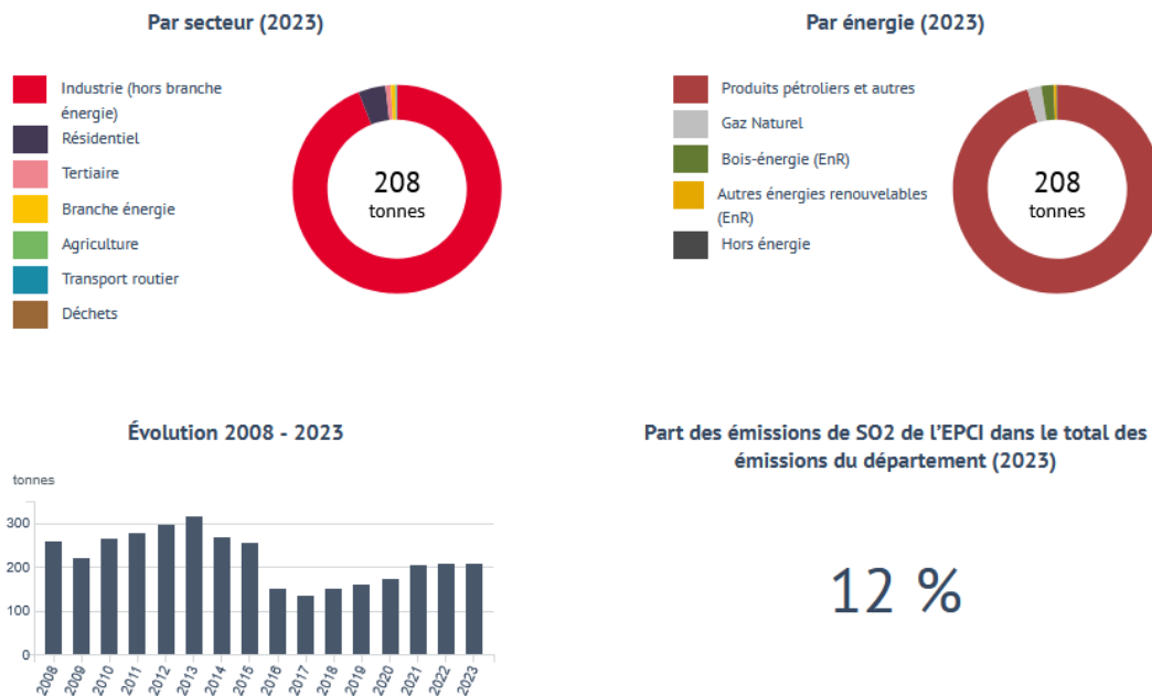
Figure 75 : Bilan des émissions de SO 2 sur la CC Châteaubriant-Derval en 2023. Source : Air Pays de la Loire
